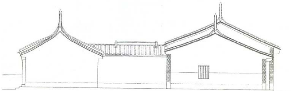
南側立面圖
