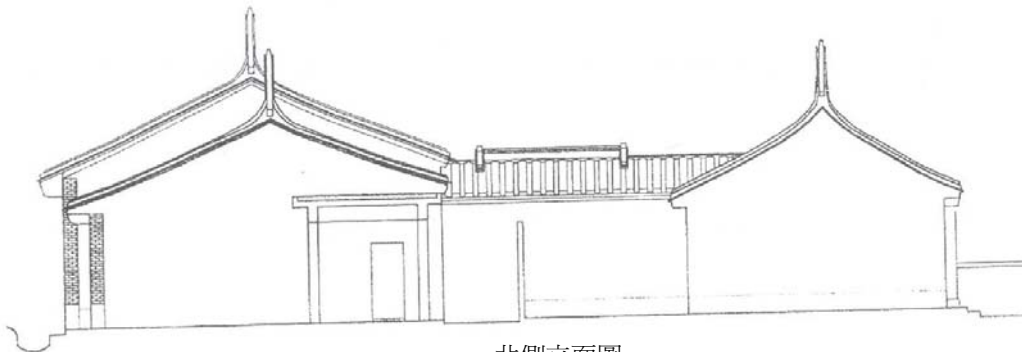
北側立面圖
