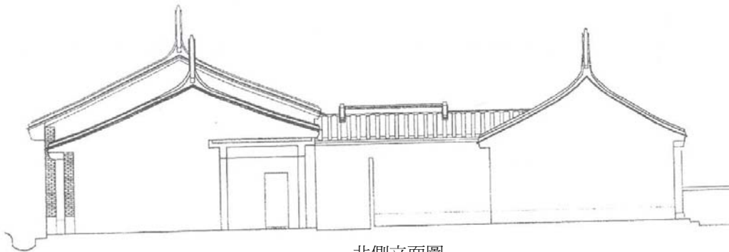
北側立面圖
