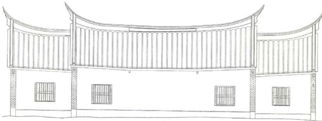
背向立面圖
