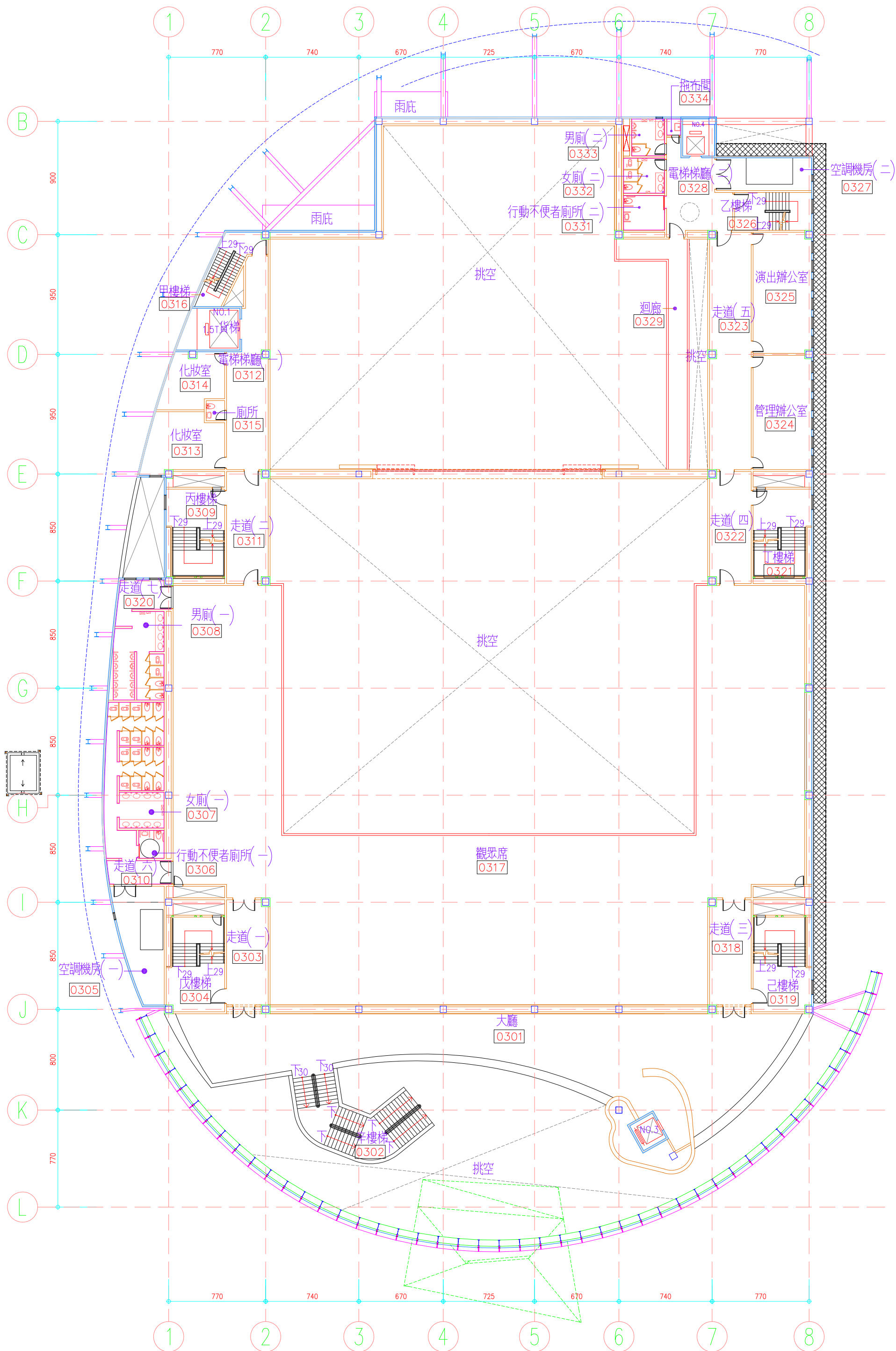
三層平面配置圖
