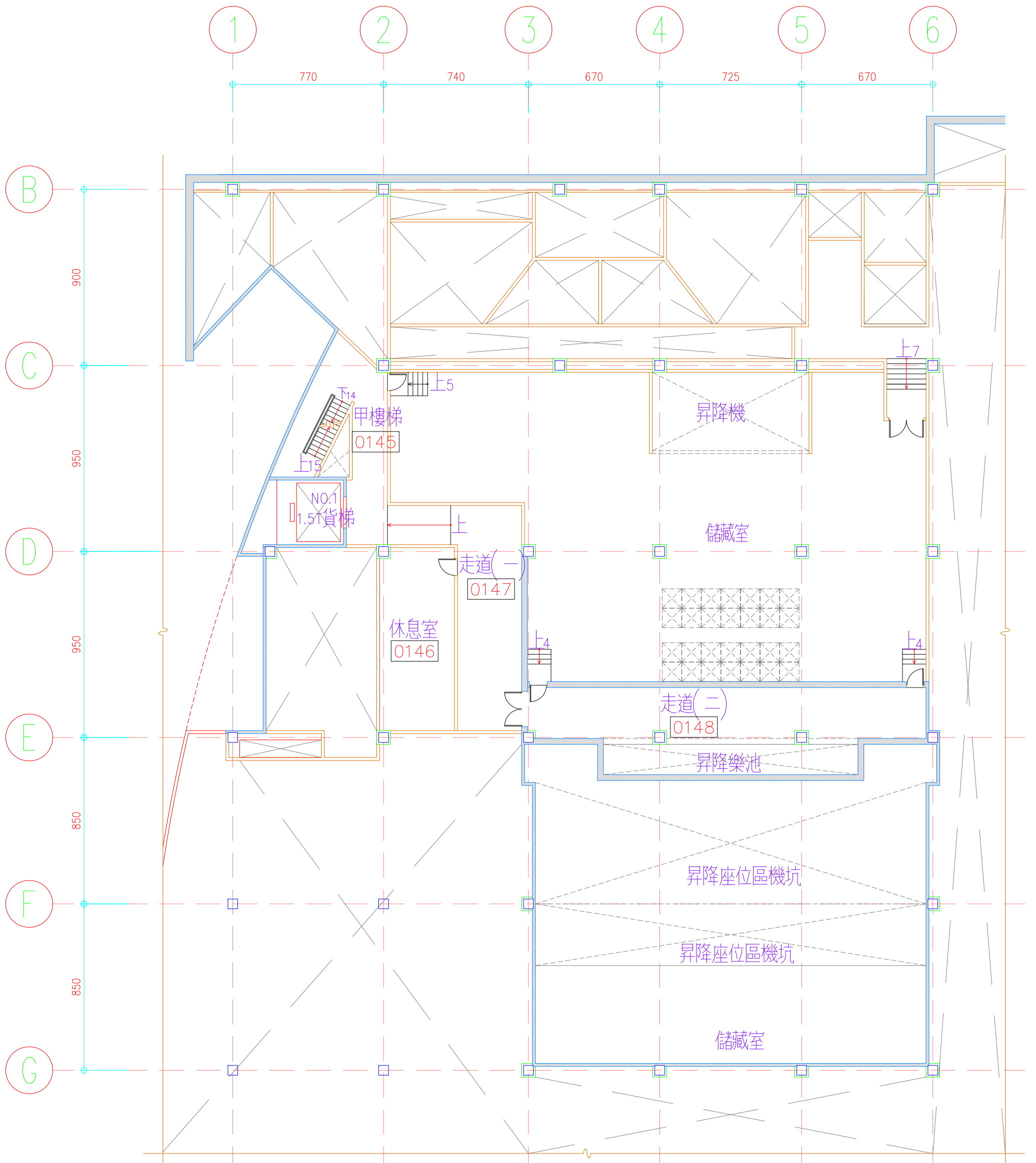
一層夾層平面配置圖
